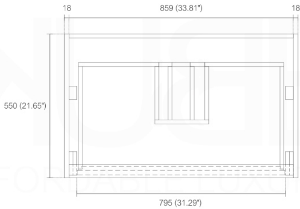
. TOP ELEVATION
